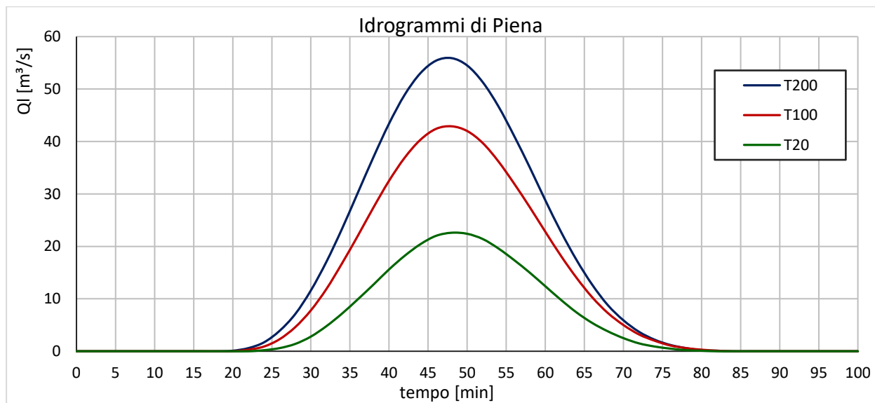
Figura 8.4: idrogramma di piena del t. Eaux Blanches per i diversi tempi di ritorno
