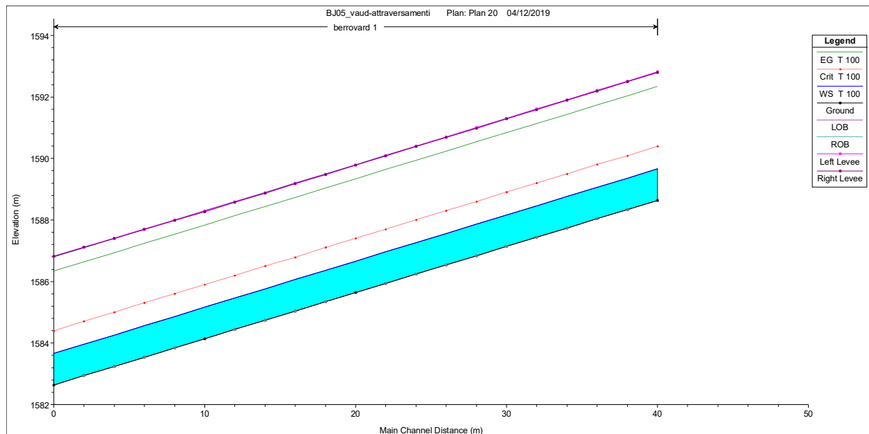
Figura 10.11: profilo per T=100 – attraversamento t. Berrovard
