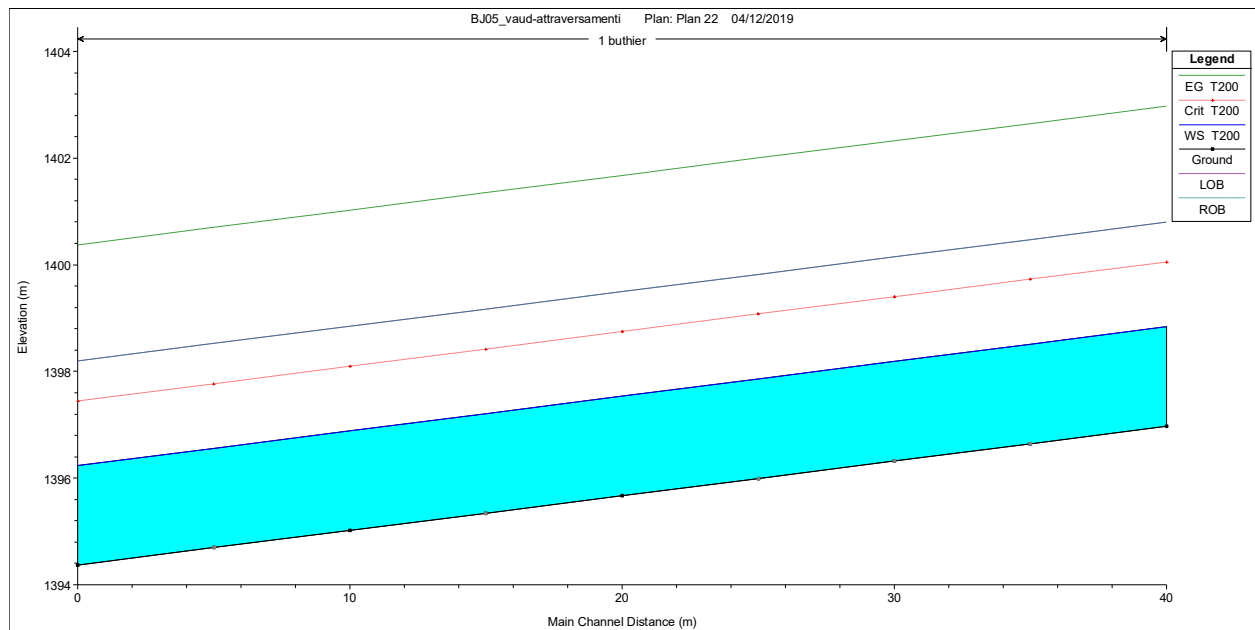
Figura 10.27: profilo per T=200 anni – Buthier scarico
