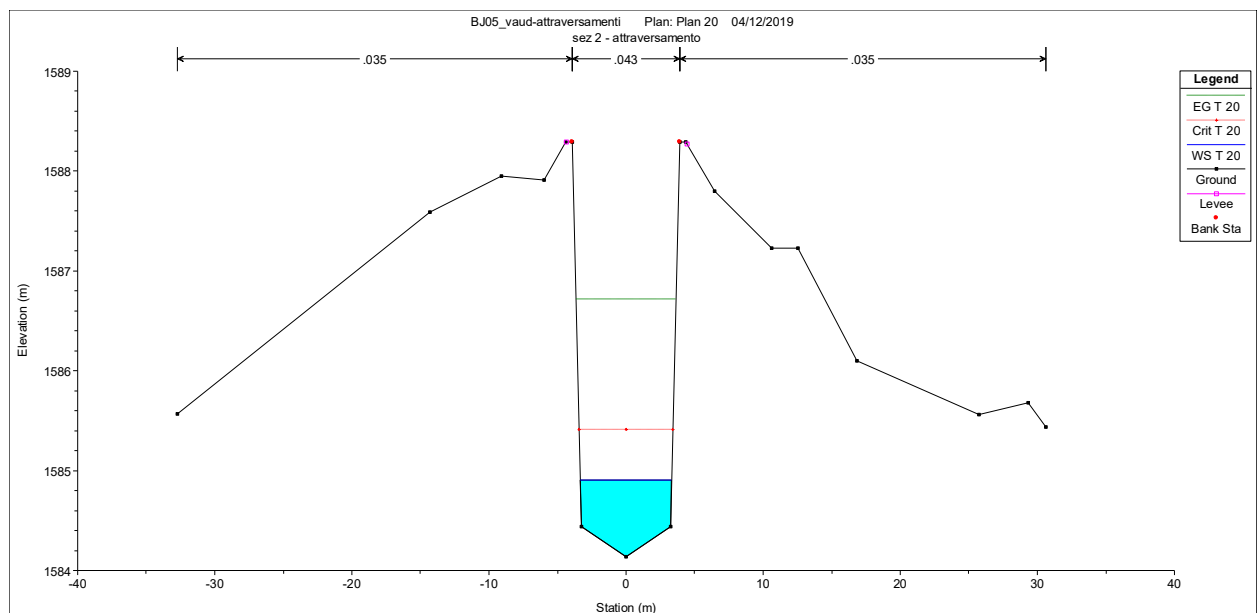
Figura 10.10: sezione attraversamento del t. Berrovard per T=20
