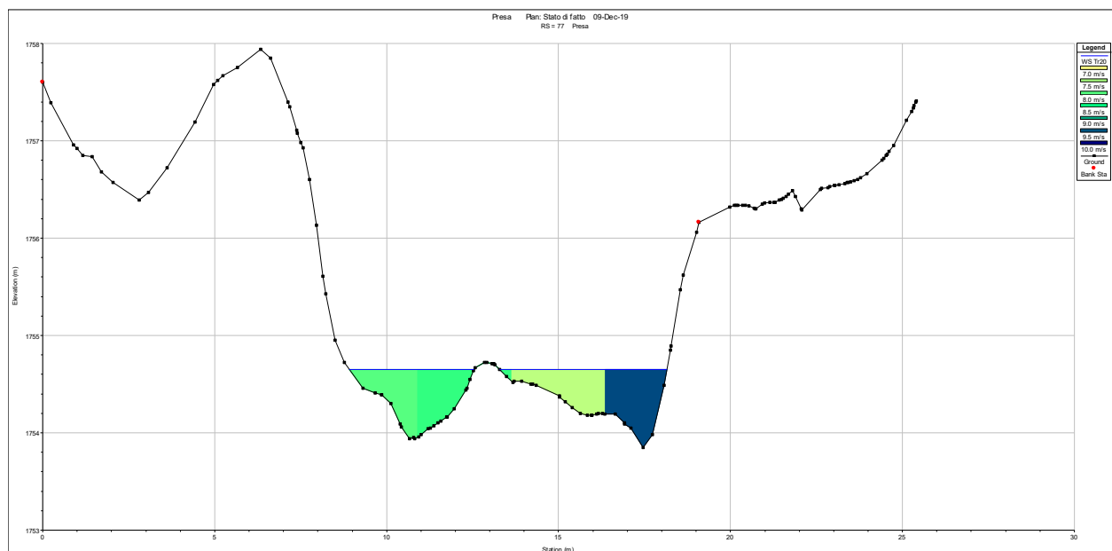
Figura 10.3: sezione della presa per T=20 – presa EauXBlanches
