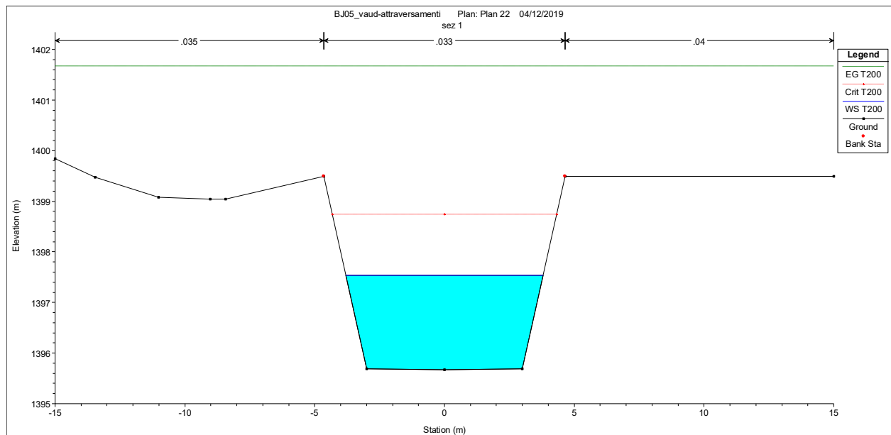
Figura 10.28: sezione del Buthier interessata dallo scarico (T=200 anni)
