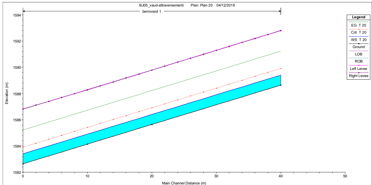
Figura 10.9: profilo per T=20 – attraversamento t. Berrovard
