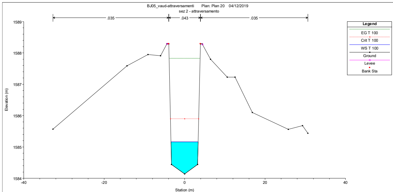
Figura 10.12: sezione attraversamento del t. Berrovard per T=100
