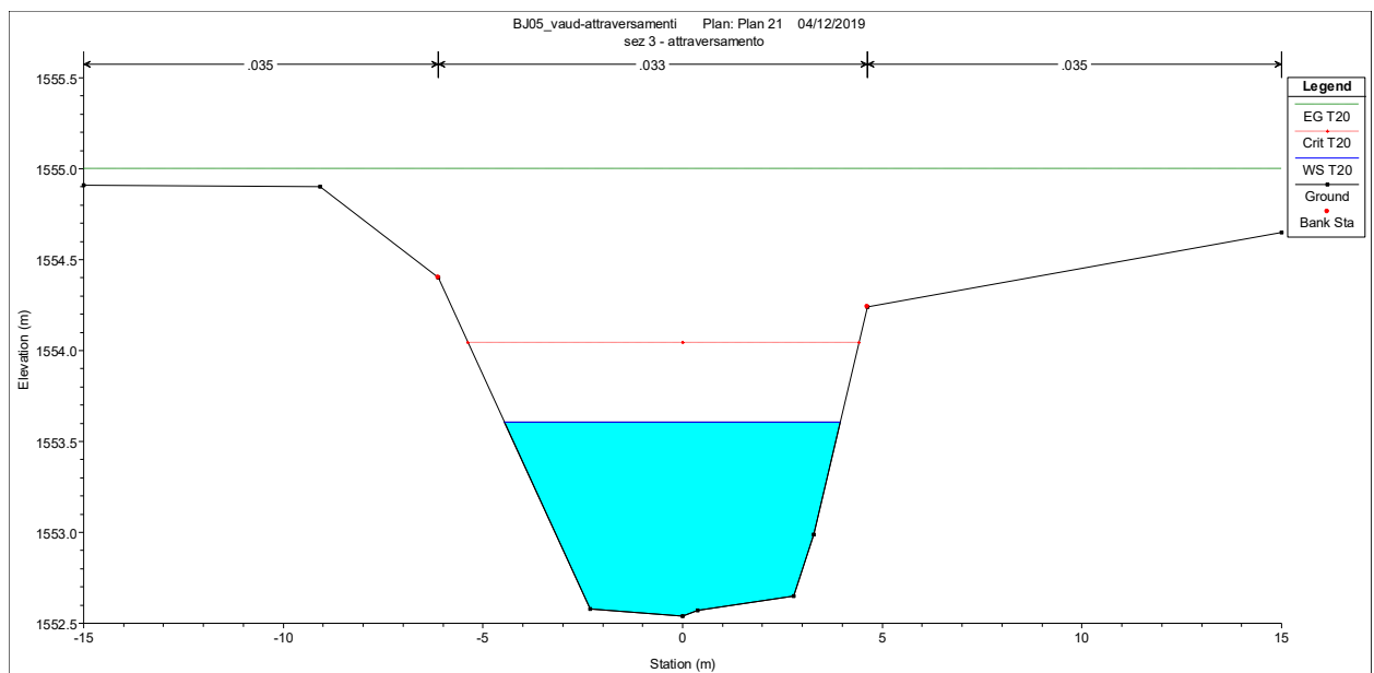
Figura 10.17: sezione attraversamento del t. Buthier per T=20
