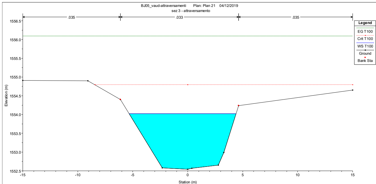
Figura 10.19: sezione attraversamento del t. Buthier per T=100
