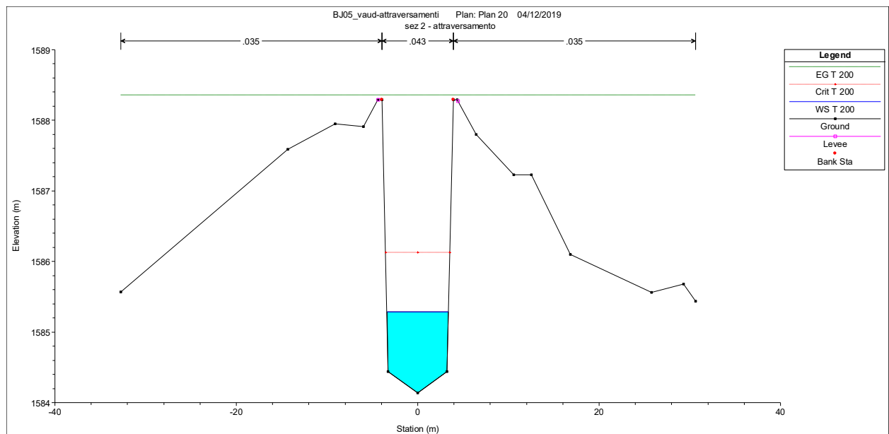
Figura 10.14: sezione attraversamento del t. Berrovard per T=200
