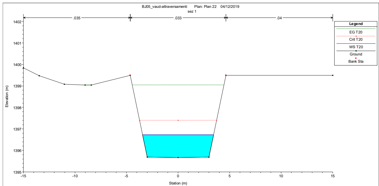
Figura 10.24: sezione del Buthier interessata dallo scarico (T=20 anni)
