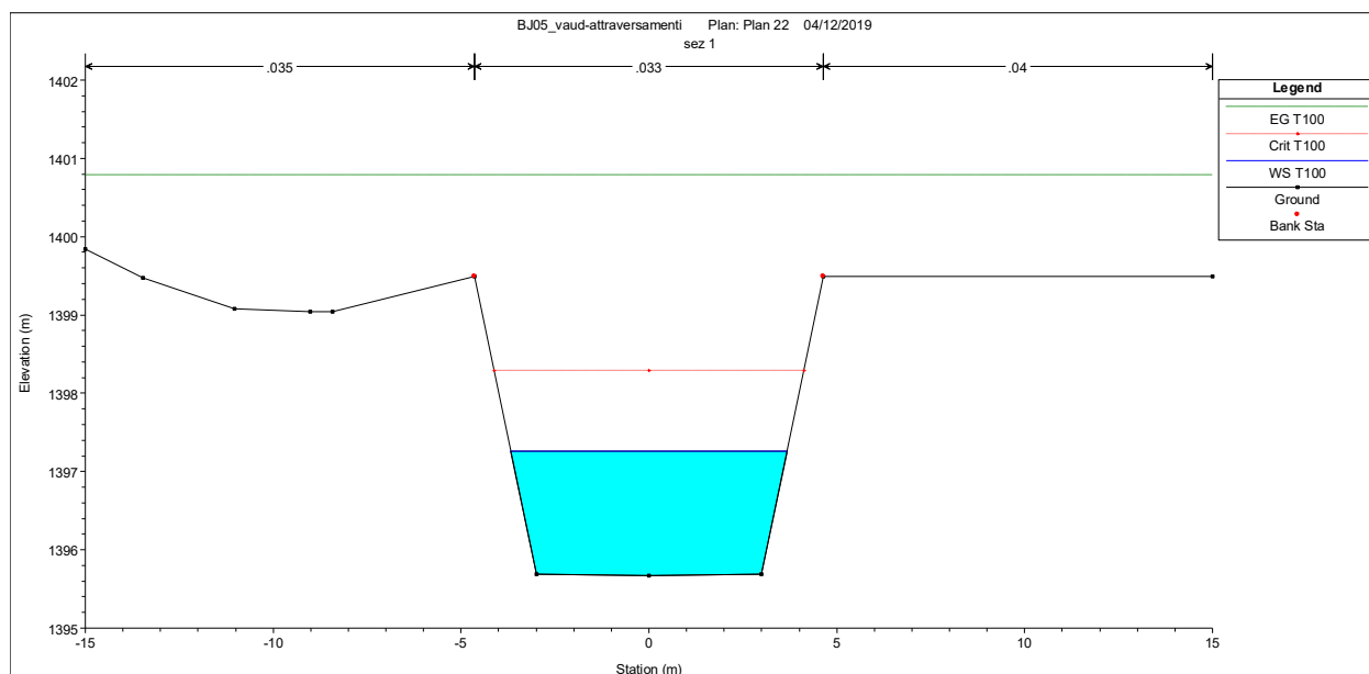
Figura 10.26: sezione del Buthier interessata dallo scarico (T=100 anni)
