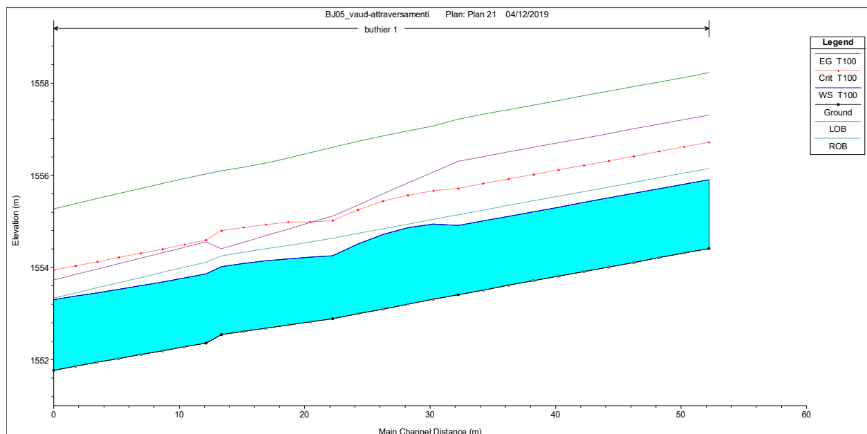
Figura 10.18: profilo idraulico per T=100 – attraversamento t. Buthier
