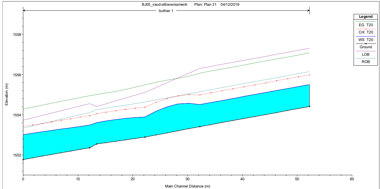
Figura 10.16: profilo idraulico per T=20 – attraversamento t. Buthier
