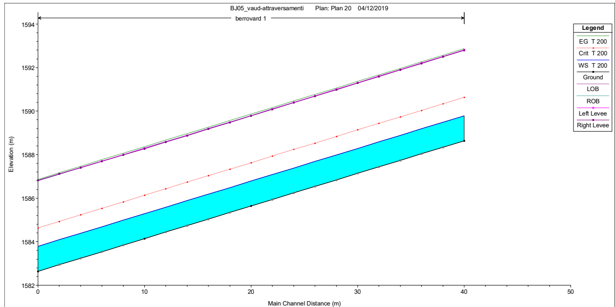
Figura 10.13: profilo per T=200 – attraversamento t. Berrovard
