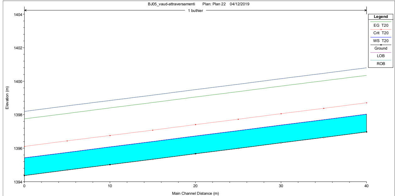
Figura 10.23: profilo per T=20 anni – Buthier scarico
