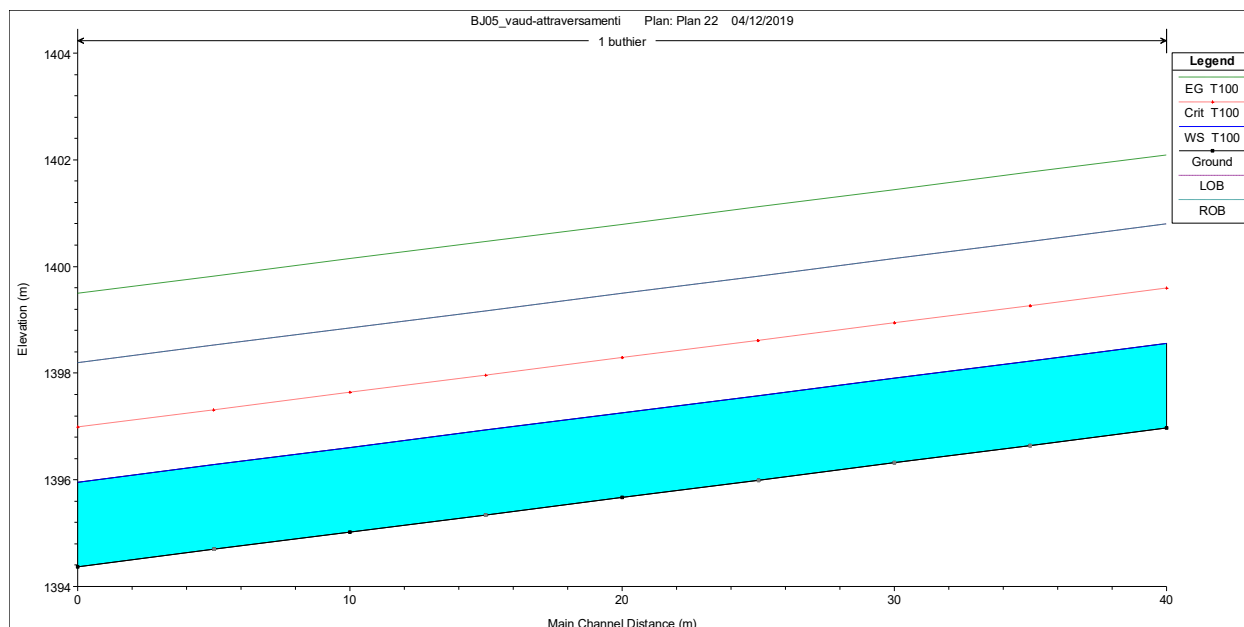
Figura 10.25: profilo per T=100 anni – Buthier scarico
