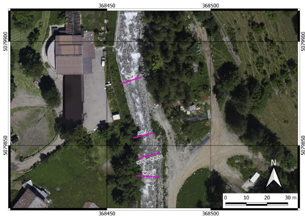
Figura 10.22: disposizione planimetrica sezioni idrauliche
