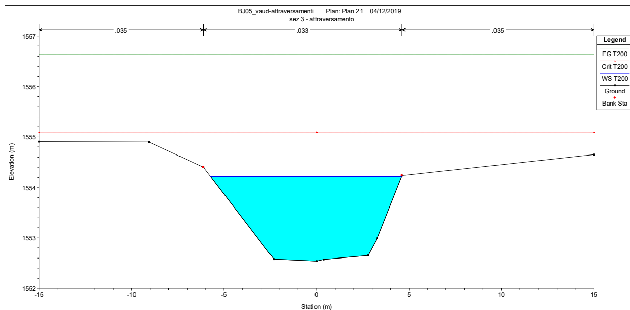
Figura 10.21: sezione attraversamento del t. Buthier per T=200
