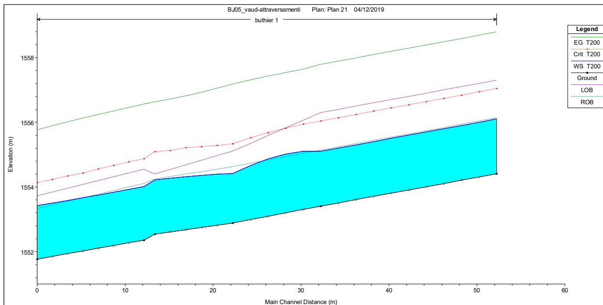
Figura 10.20: profilo idraulico per T=200 – attraversamento t. Buthier
